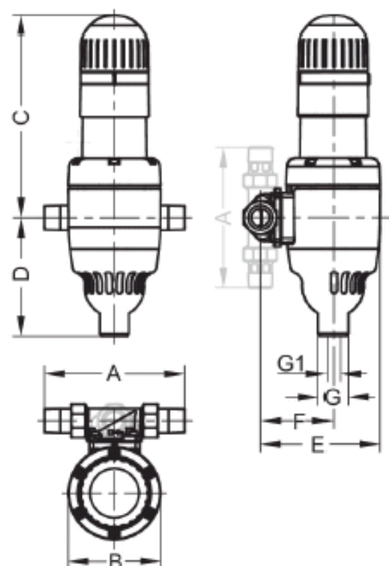
Fig. : JPF+ 3/4" - 1 1/4"
